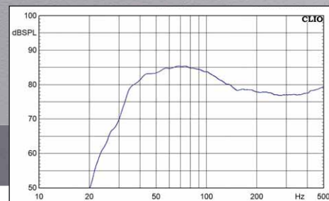
Der MWS822 schöpft in 17 Litern aus dem Vollen. Mit einer tiefen Abstimmung erreicht er die 40 Hz Marke
