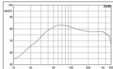
Der MWS1022 läuft im geschlossenen Gehäuse zwar nur mit 83 dB an 1 W, dafür spielt er gleichmäßig und sauber bis in den Tiefbass
